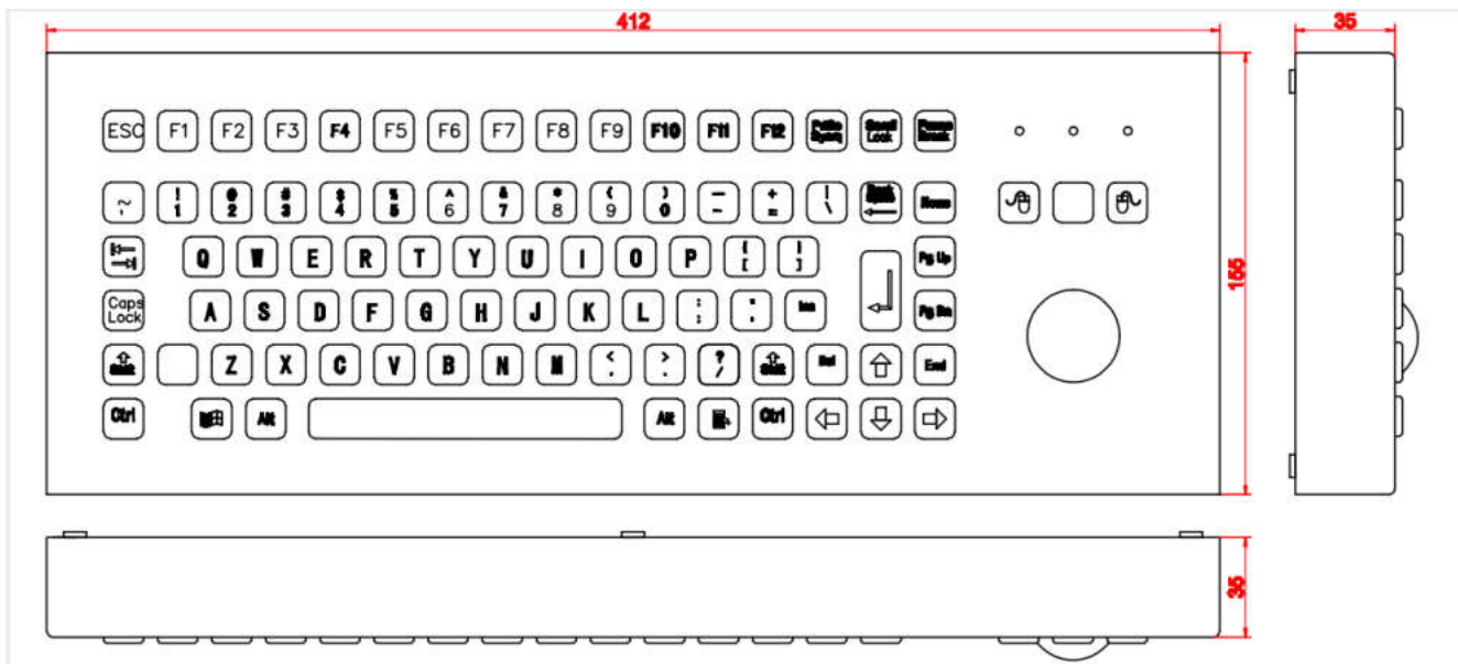
尺寸图
