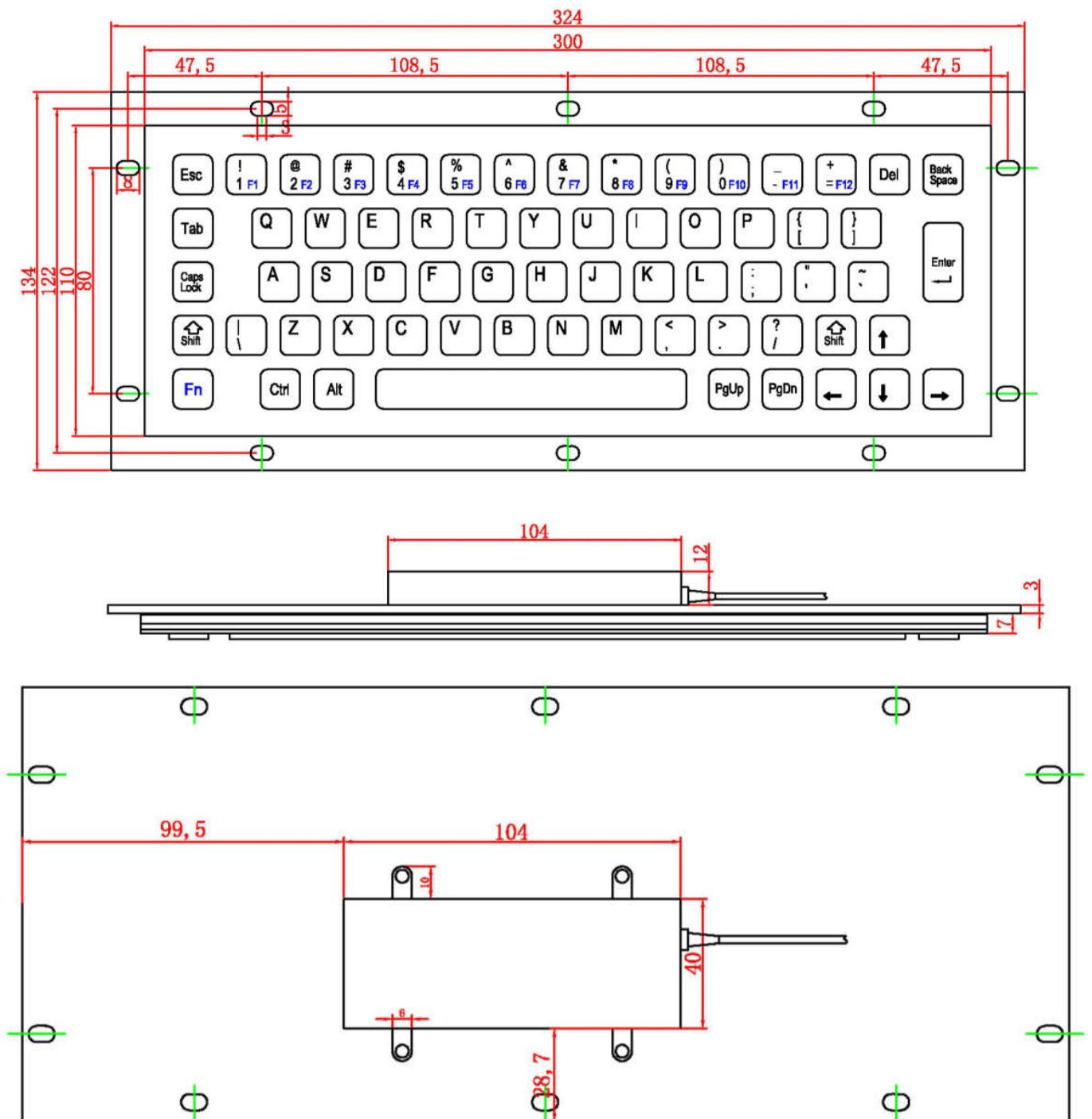
尺寸图
