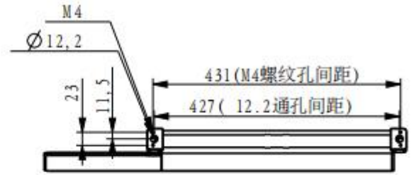
A视图(安装尺寸图)
