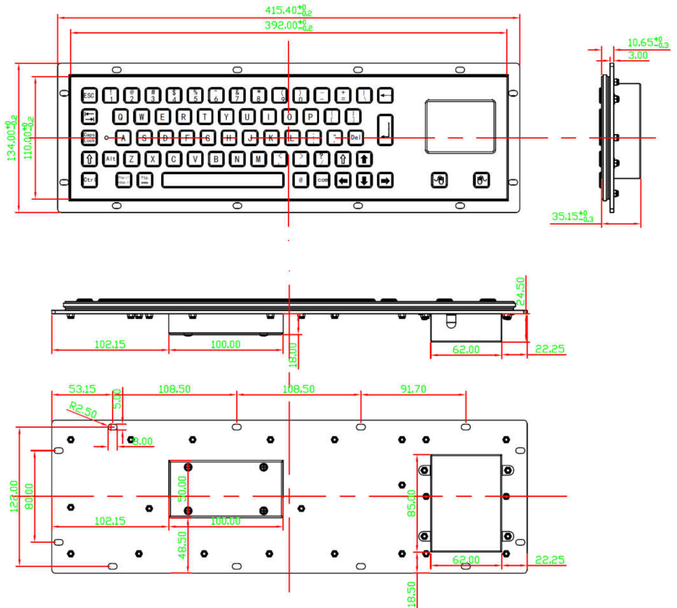
尺寸图
