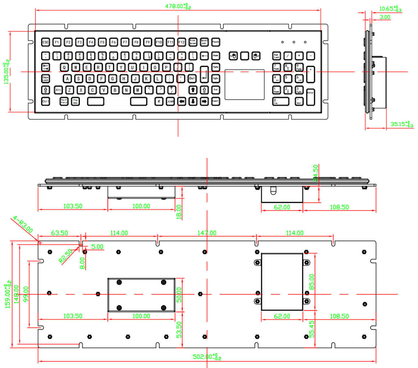
尺寸图
