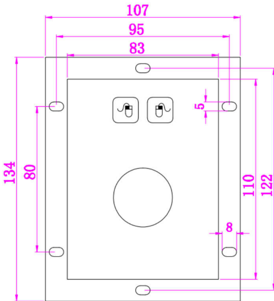
尺寸图
